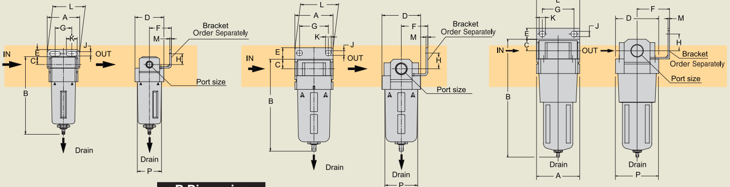
Size FA2
